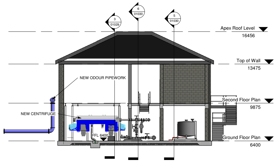
4 Section 2 1 : 100
